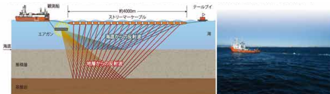
弾性波探査の概念図
